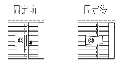
グレーチング固定部詳細図
