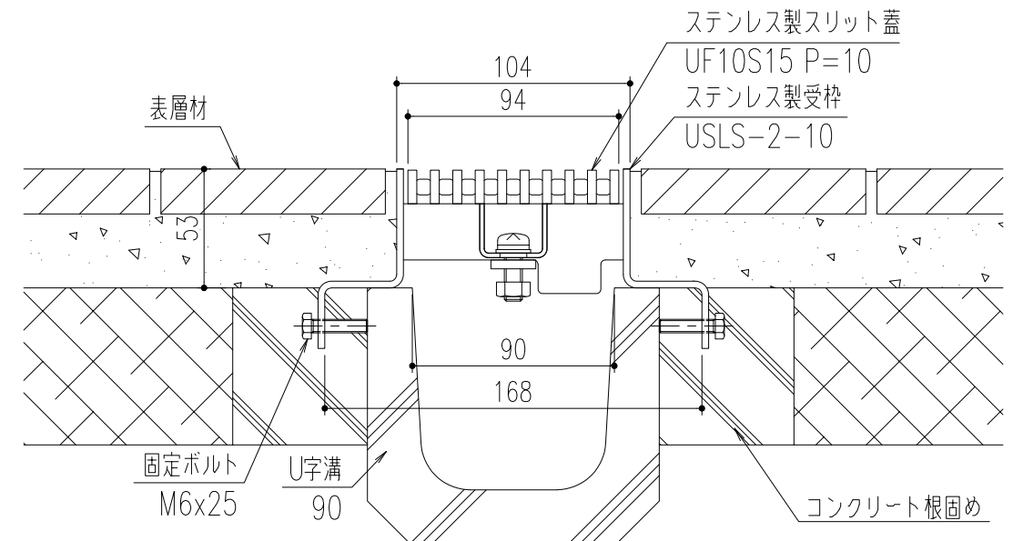
納まり断面図 (S=1/3)
