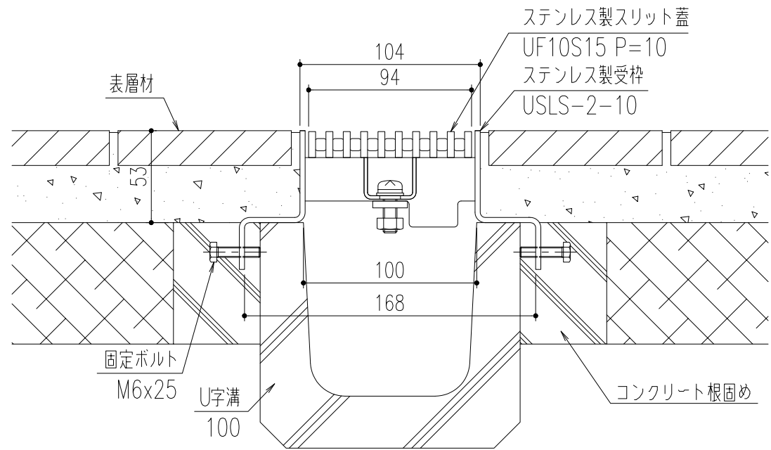
納まり断面図 (S=1/3)
