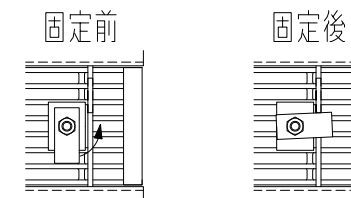
グレーチング固定部詳細図
