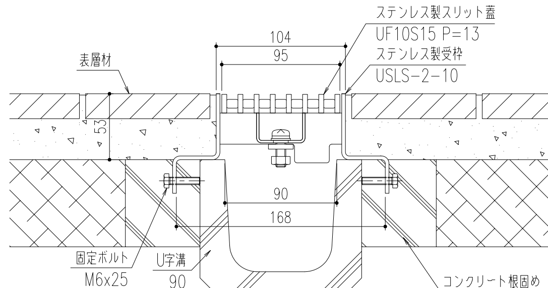
納まり断面図 (S=1/3)
