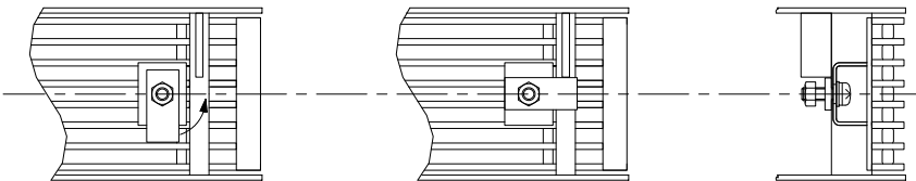
グレーチング固定部詳細図
