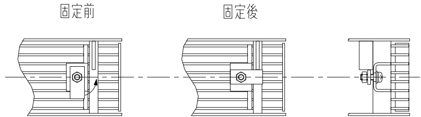
グレーチング固定部詳細図
