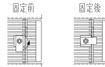
グレーチング固定部詳細図
