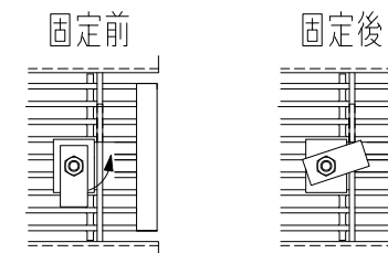
グレーチング固定部詳細図
