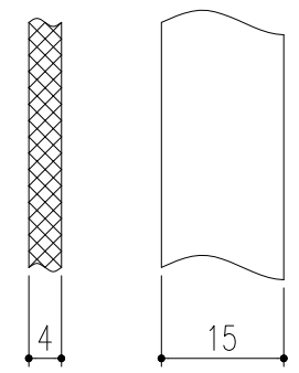
ベアリングバー詳細図
