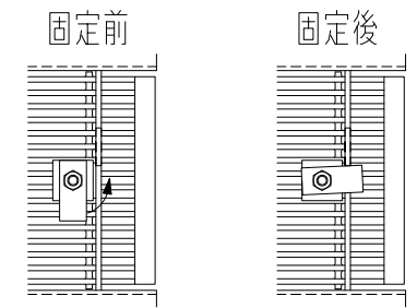
グレーチング固定部詳細図
