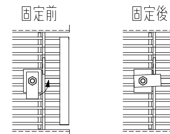
グレーチング固定部詳細図
