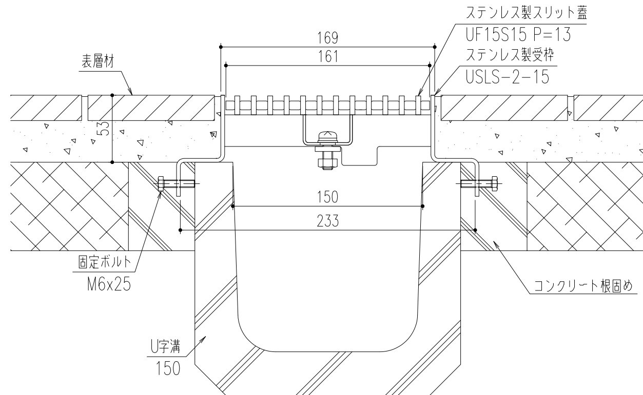
納まり断面図 (S=1/3)
