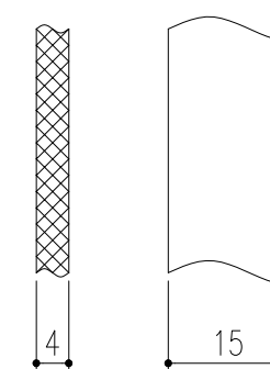
ベアリングバー詳細図
