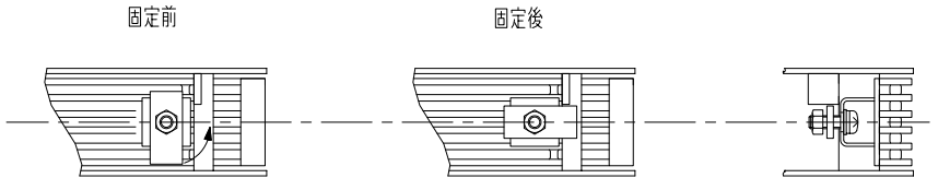
グレーチング固定部詳細図
