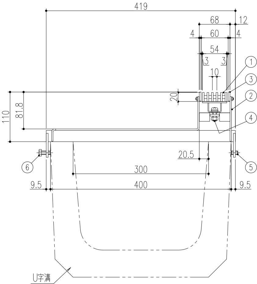
ベアリングバー詳細図
