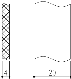
ベアリングバー詳細図
