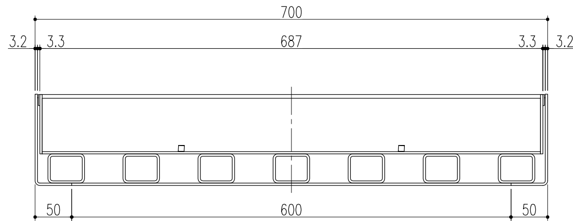
矢視B 断面図
