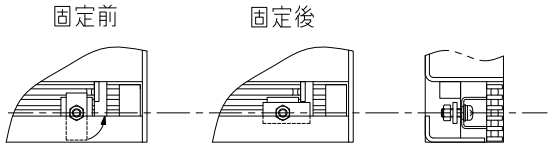
グレーチング固定部詳細図
