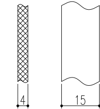
ベアリングバー詳細図
