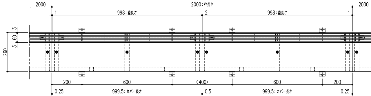
平面詳細図 S=1/10
