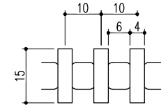
蓋詳細図 S=1/1
