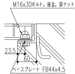
ボルト固定 詳細図
