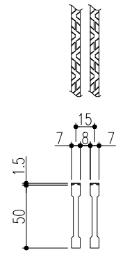
ベアリングバー 詳細図
