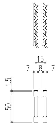
ベアリングバー 詳細図
