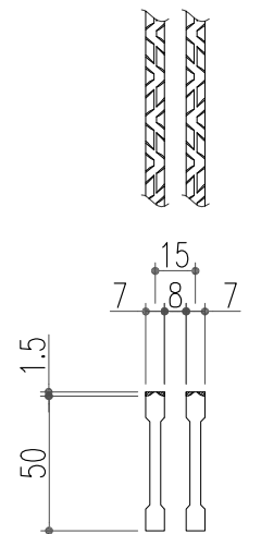
ベアリングバー 詳細図
