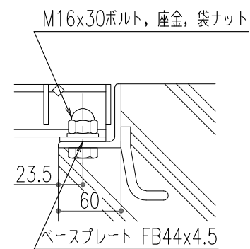
ボルト固定 詳細図
