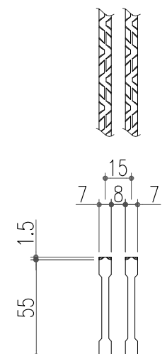
ベアリングバー 詳細図
