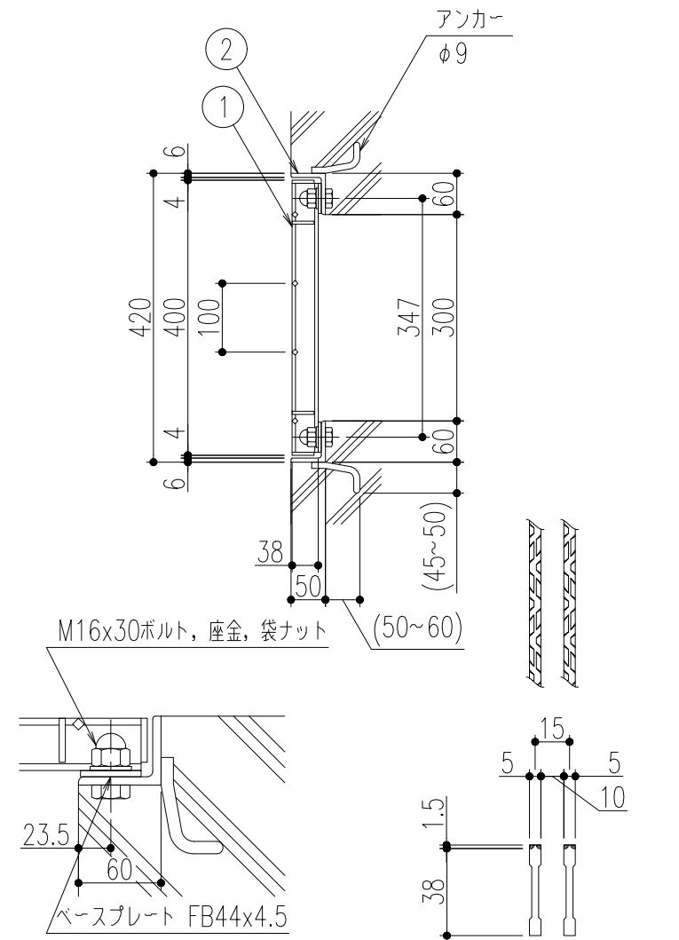
ボルト固定 詳細図
