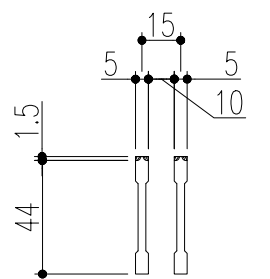
ベアリングバー 詳細図
