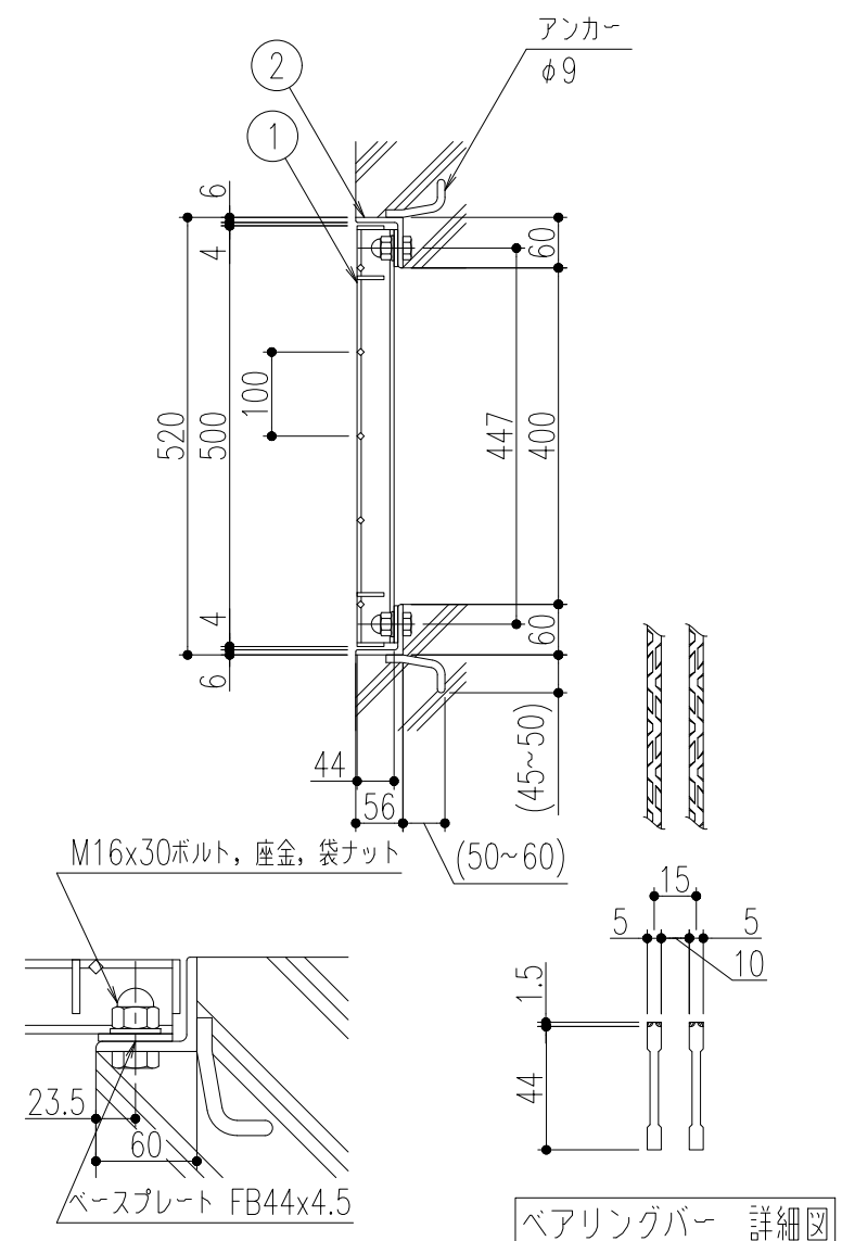
ボルト固定 詳細図
