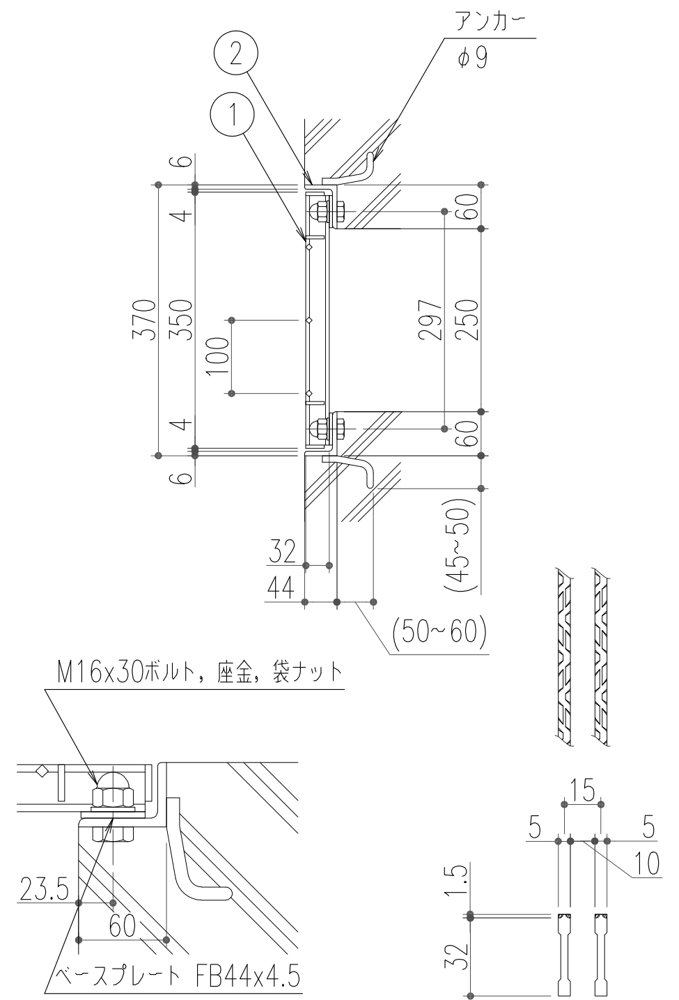
ボルト固定 詳細図
