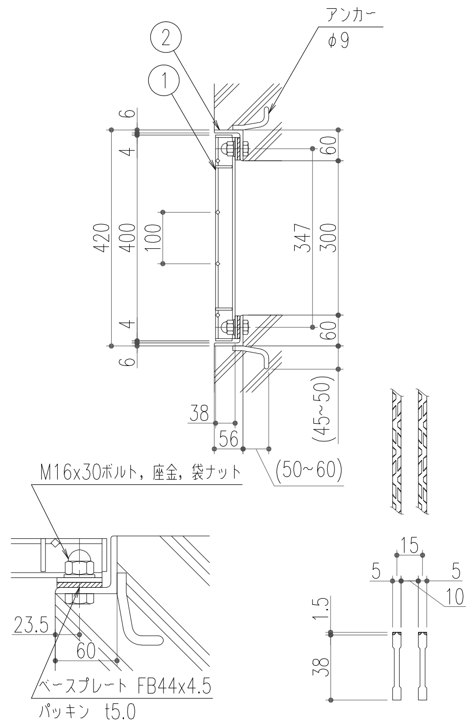
ベアリングバー 詳細図
