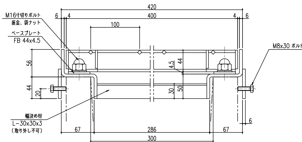
断面詳細図 S= 1/3
