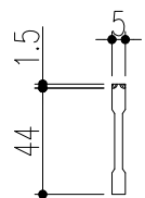
ベアリングバー 詳細図
