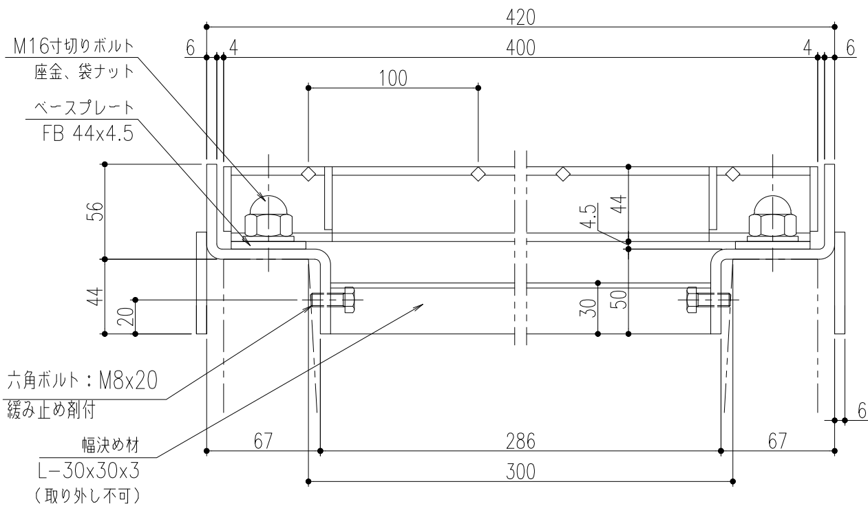
断面詳細図 S= 1/3
