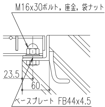
ボルト固定 詳細図
