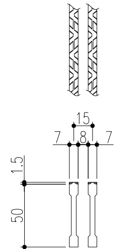
ベアリングバー 詳細図
