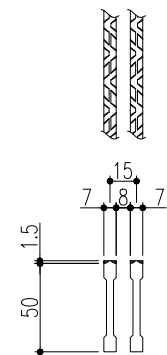
ベアリングバー 詳細図
