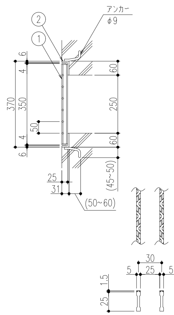
ベアリングバー 詳細図
