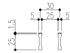
ベアリングバー 詳細図
