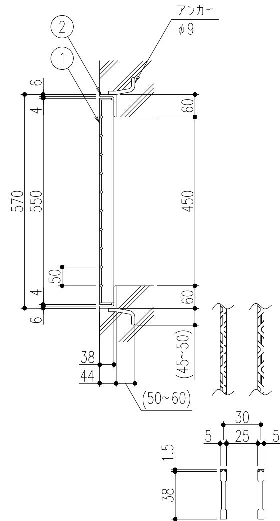
ベアリングバー 詳細図
