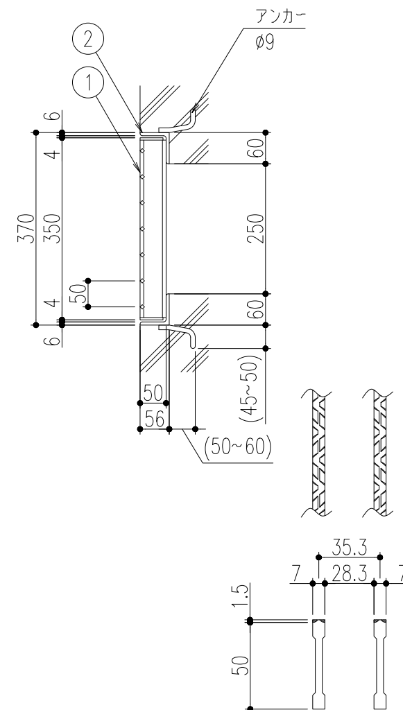
ベアリングバー 詳細図
