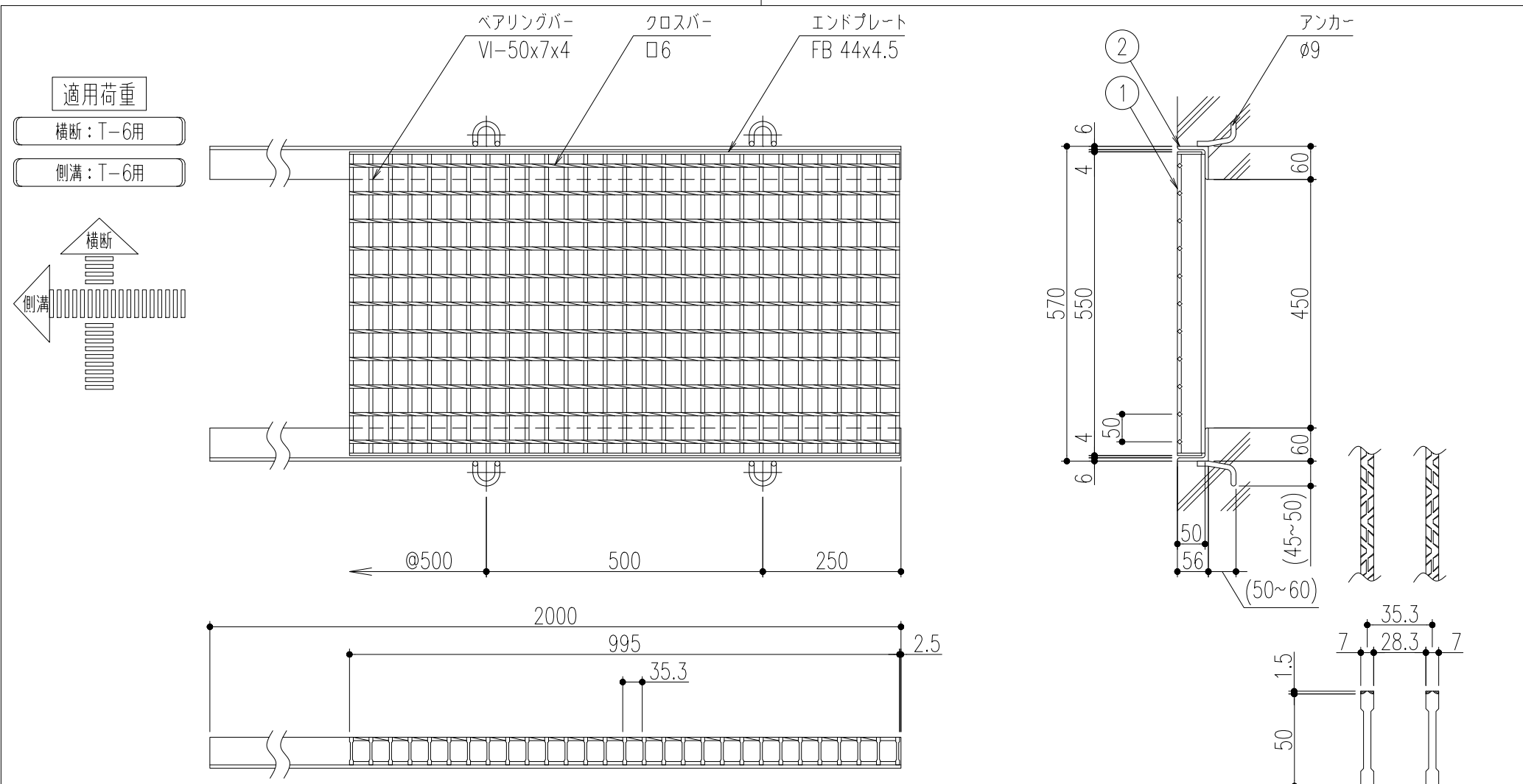
ベアリングバー 詳細図
