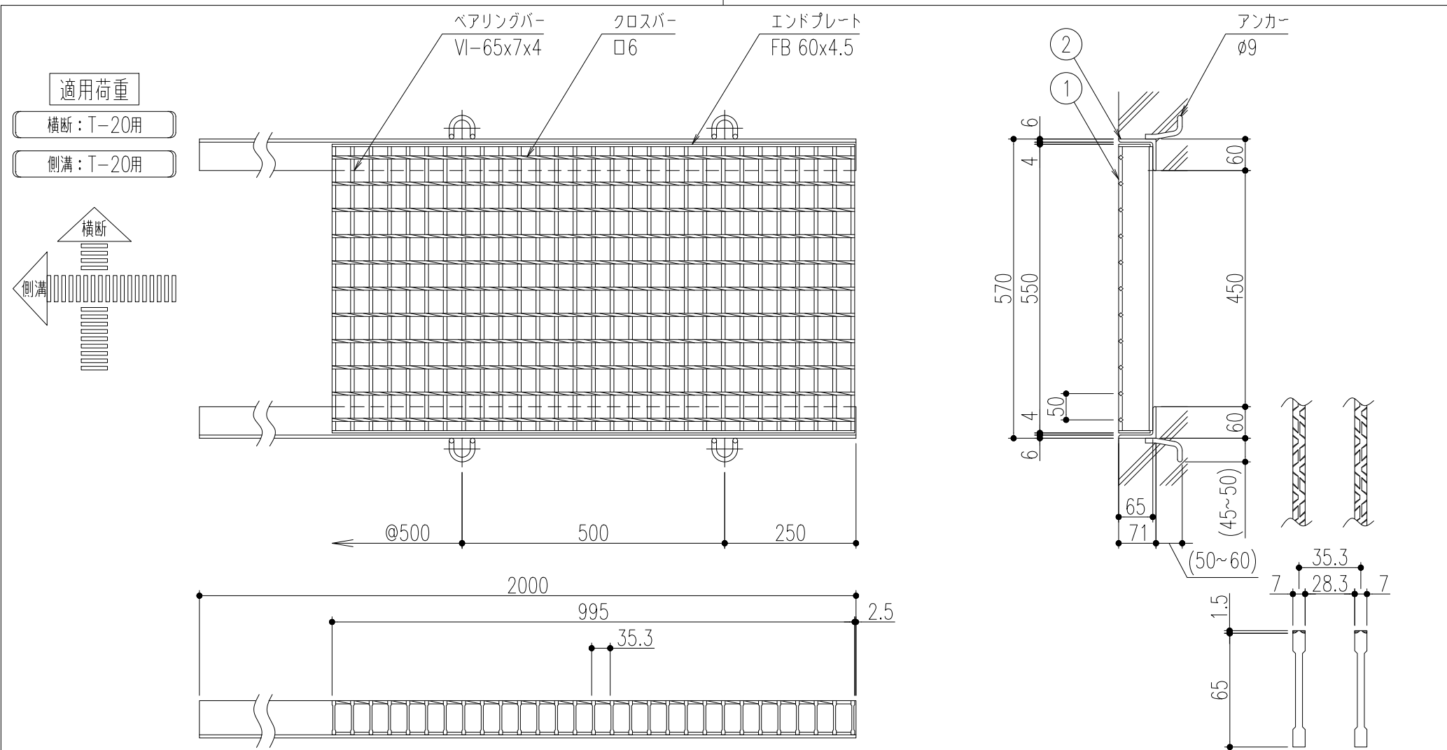
ベアリングバー 詳細図
