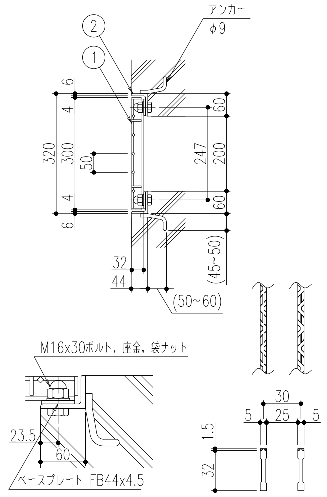
ボルト固定 詳細図
