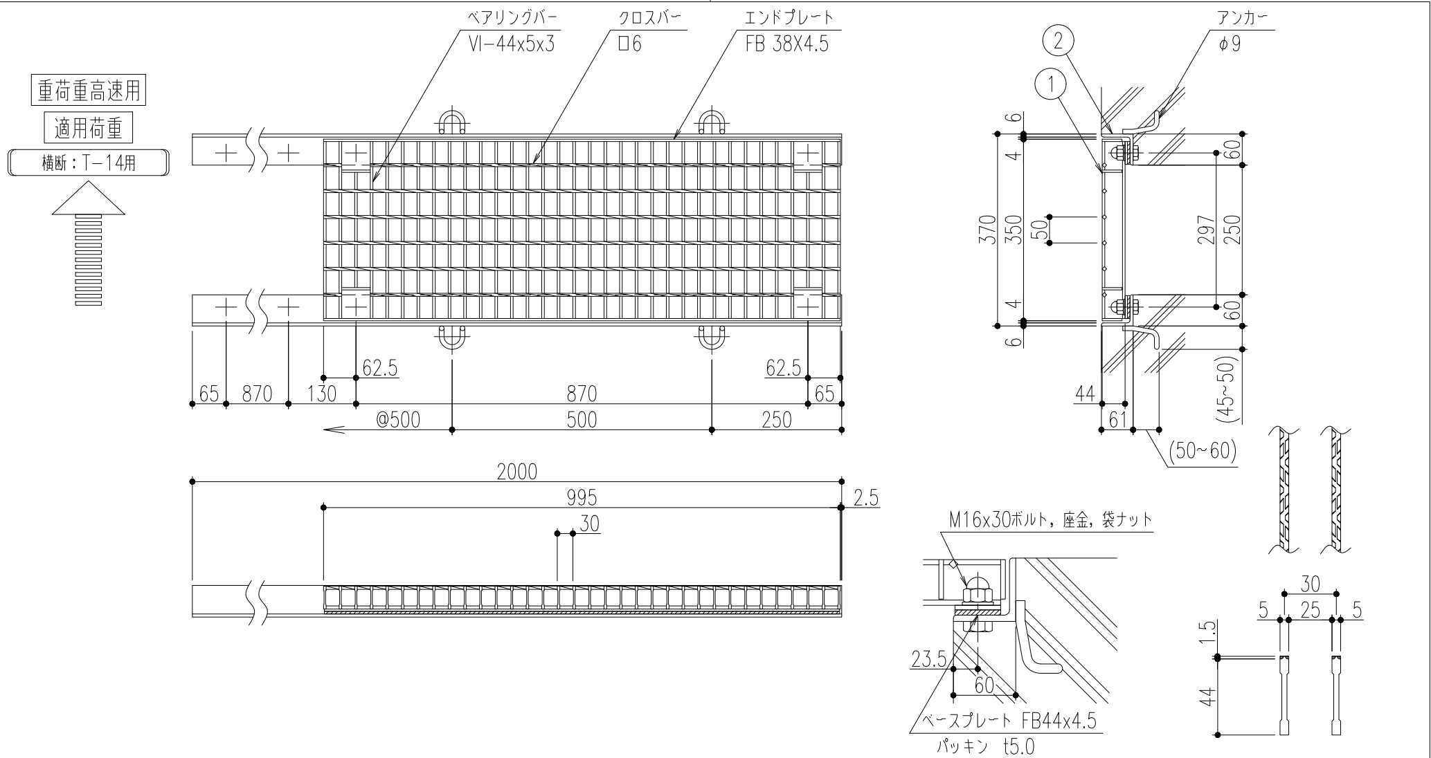
ボルト固定 詳細図
