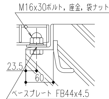
ボルト固定 詳細図
