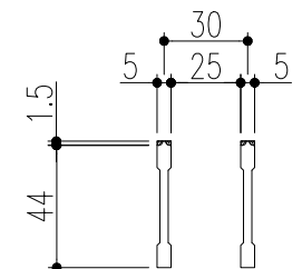
ベアリングバー 詳細図
