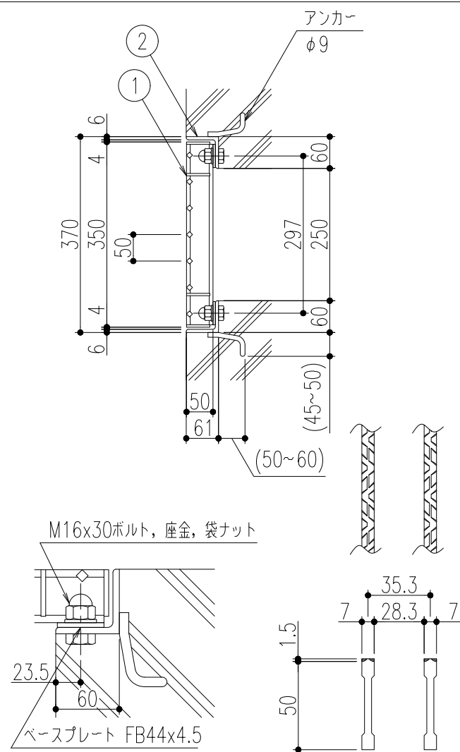
ボルト固定 詳細図
