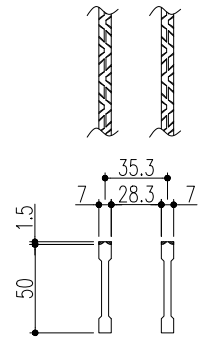
ベアリングバー 詳細図
