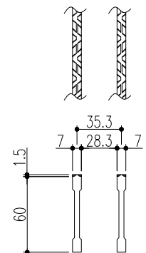
ベアリングバー 詳細図
