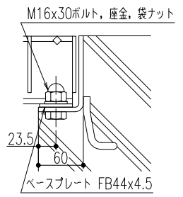
ボルト固定 詳細図
