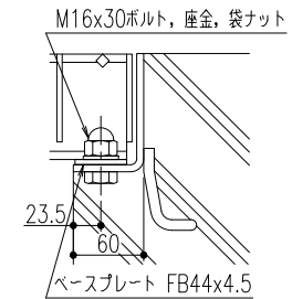
ボルト固定 詳細図
