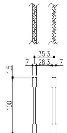
ベアリングバー 詳細図
