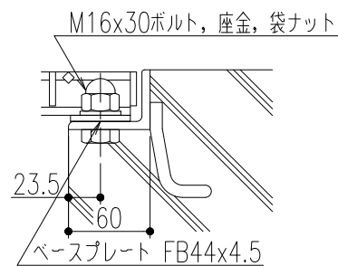
ボルト固定 詳細図
