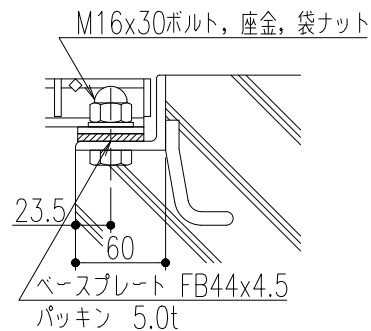
ボルト固定 詳細図
