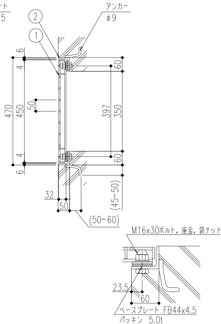
ボルト固定 詳細図
