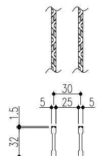
ベアリングバー 詳細図
