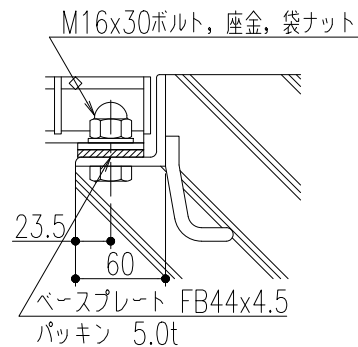
ボルト固定 詳細図
